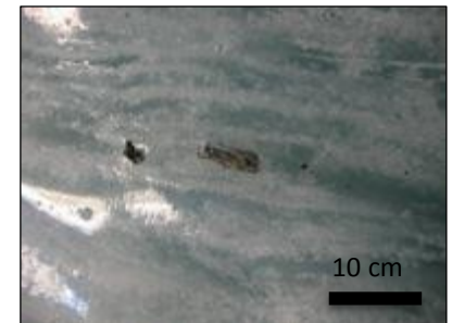
Abbildung 5: Eiskaverne im Mer de Glace Gletscher, Chamonix: Das Eis erscheint durch Bänder mit Luftblasen (weiss) und Gesteinstrümmern (dunkel) geschichtet.
