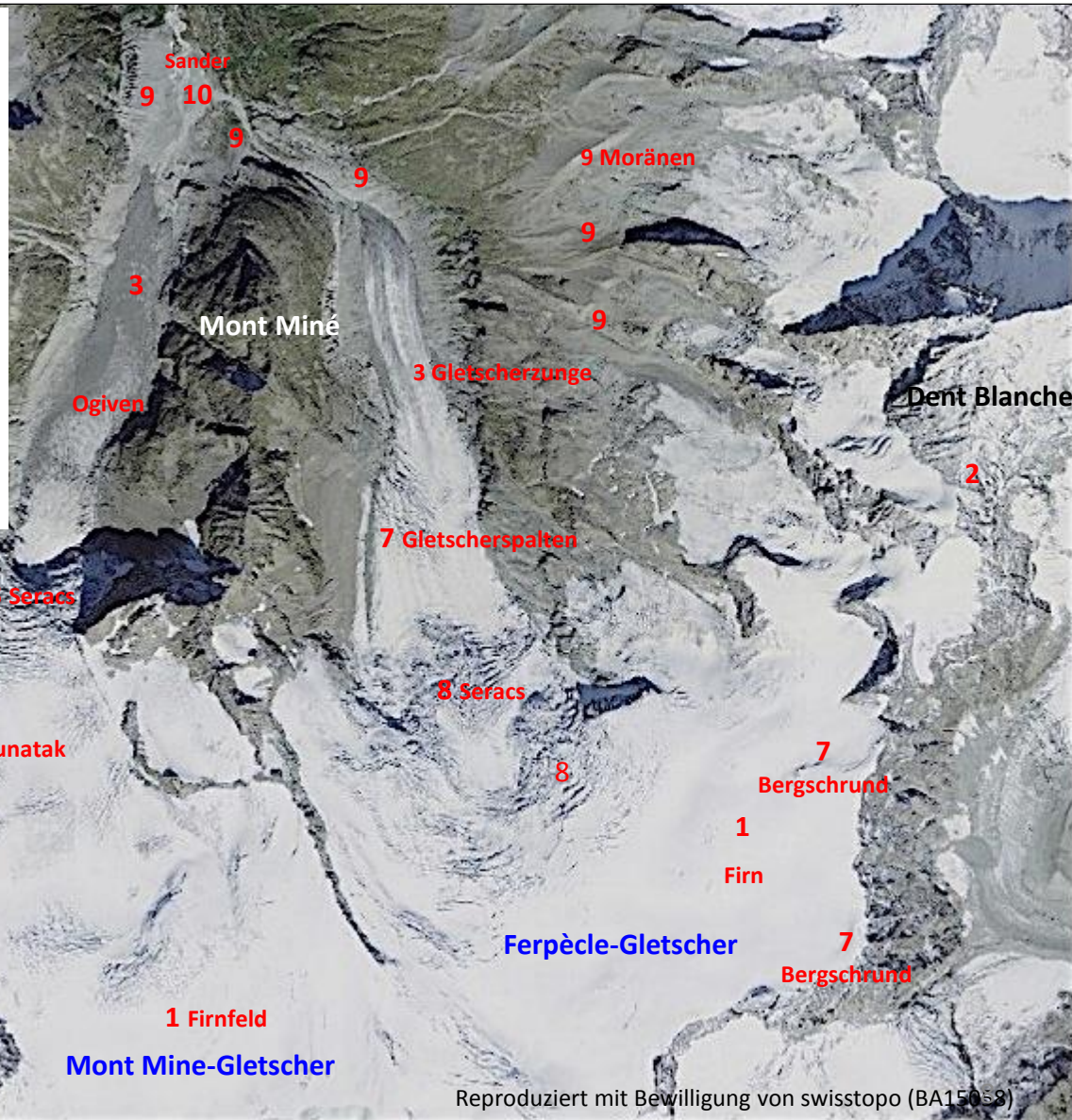
Abbildung 11: Gazialsystem der Gletscher von Mont Miné und Ferpèche
