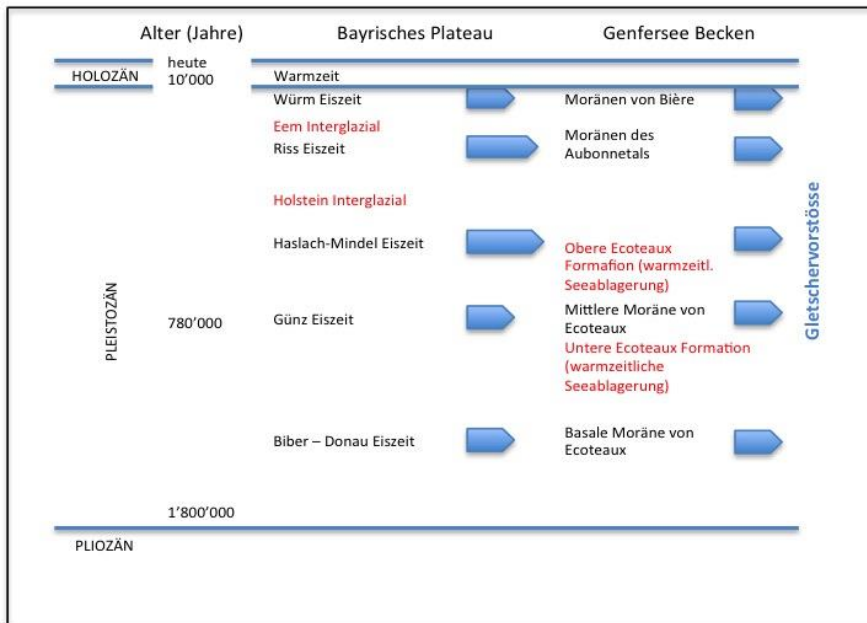
Abbildung 41: Eiszeiten im Rhonetal und im Genfersee Gebiet: Vergleich mit dem Bayrischen Plateau der Ostalpen, der Typusregion der alpinen Eiszeiten (vereinfacht nach Lih et al. 2002, Genfersee Becken: Pugin et al. 1993)
