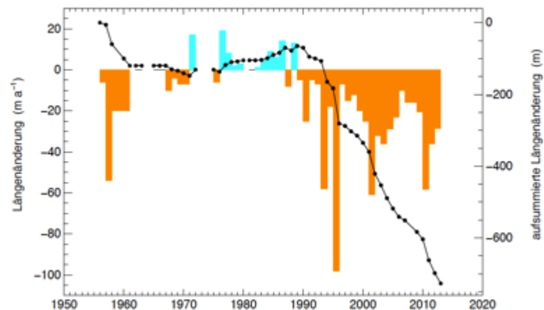
Abbildung 61: Mont Mine-Gletscher, Längenänderungen 1956 – 2013*. Schwarz: Kumulierte Länge der Veränderungen.
