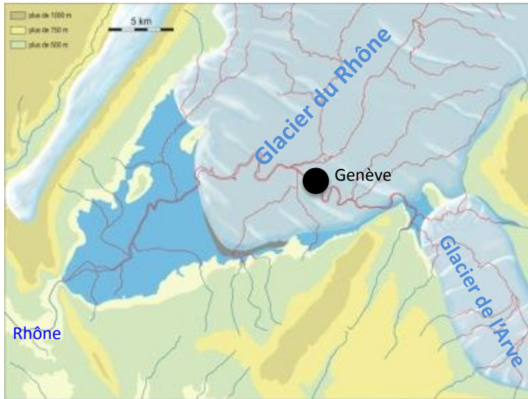
Abbildung 44: Letztes Maximum des Rhonegletschers im Genferseebecken bei Laconnex, 8 km westlich Genf, vor etwa 23'500 Jahren. Das Niveau des Seespiegels liegt bei etwa 450 m Höhe (Wildi et al. 2014).
